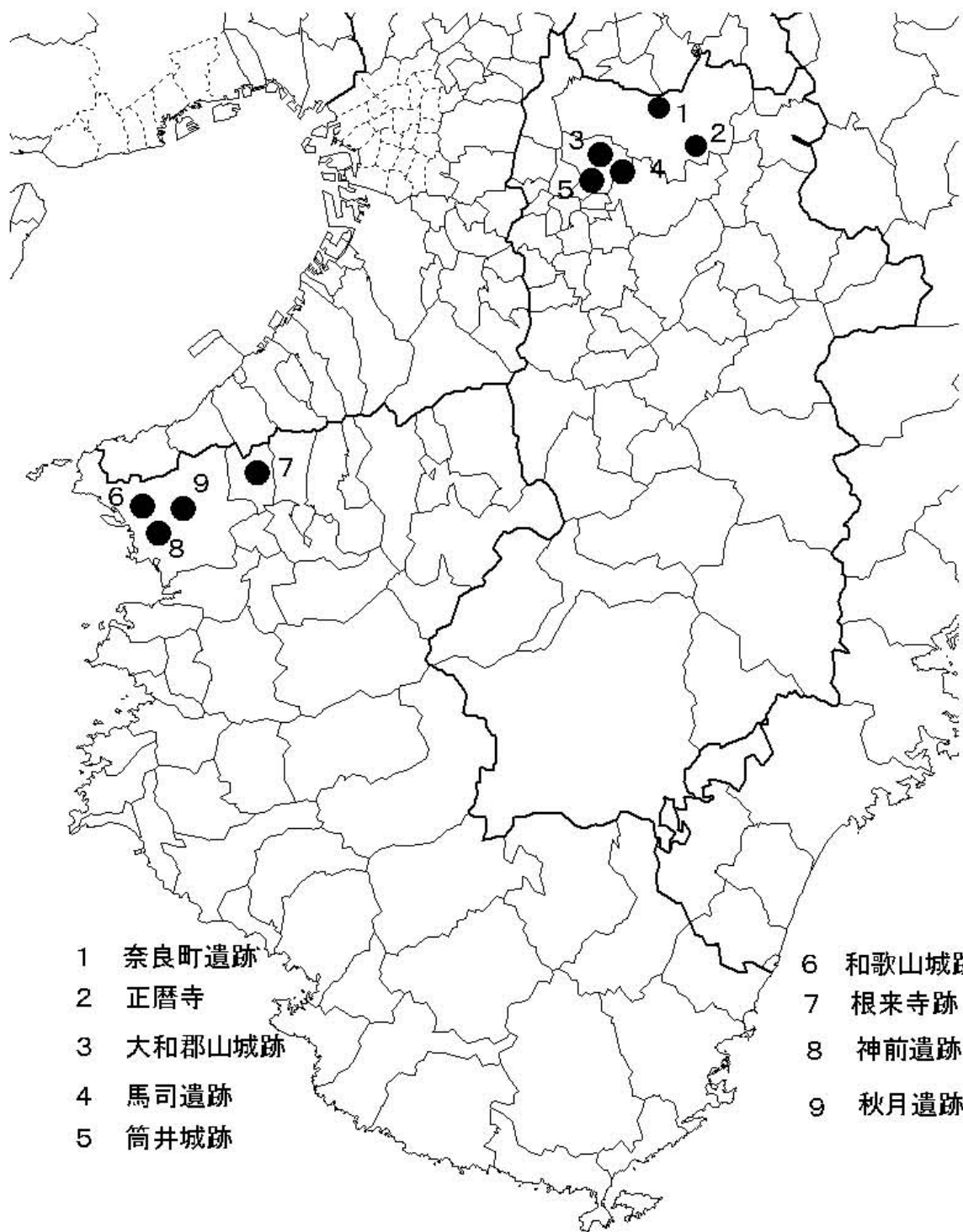
第36図 和歌山・奈良県遺跡位置図 S=1/800.000
