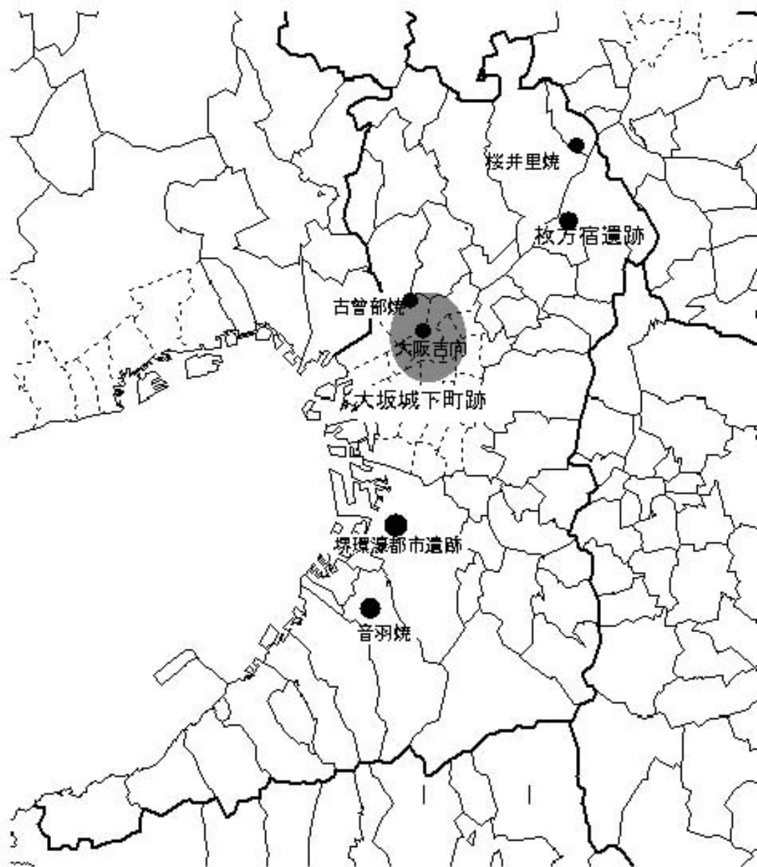
第67図 大阪府下京焼系陶器窯分布図 S=1/500,000
